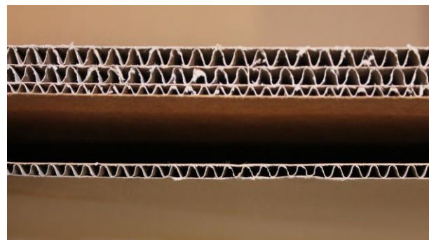
Innenhülle 3-wellig
